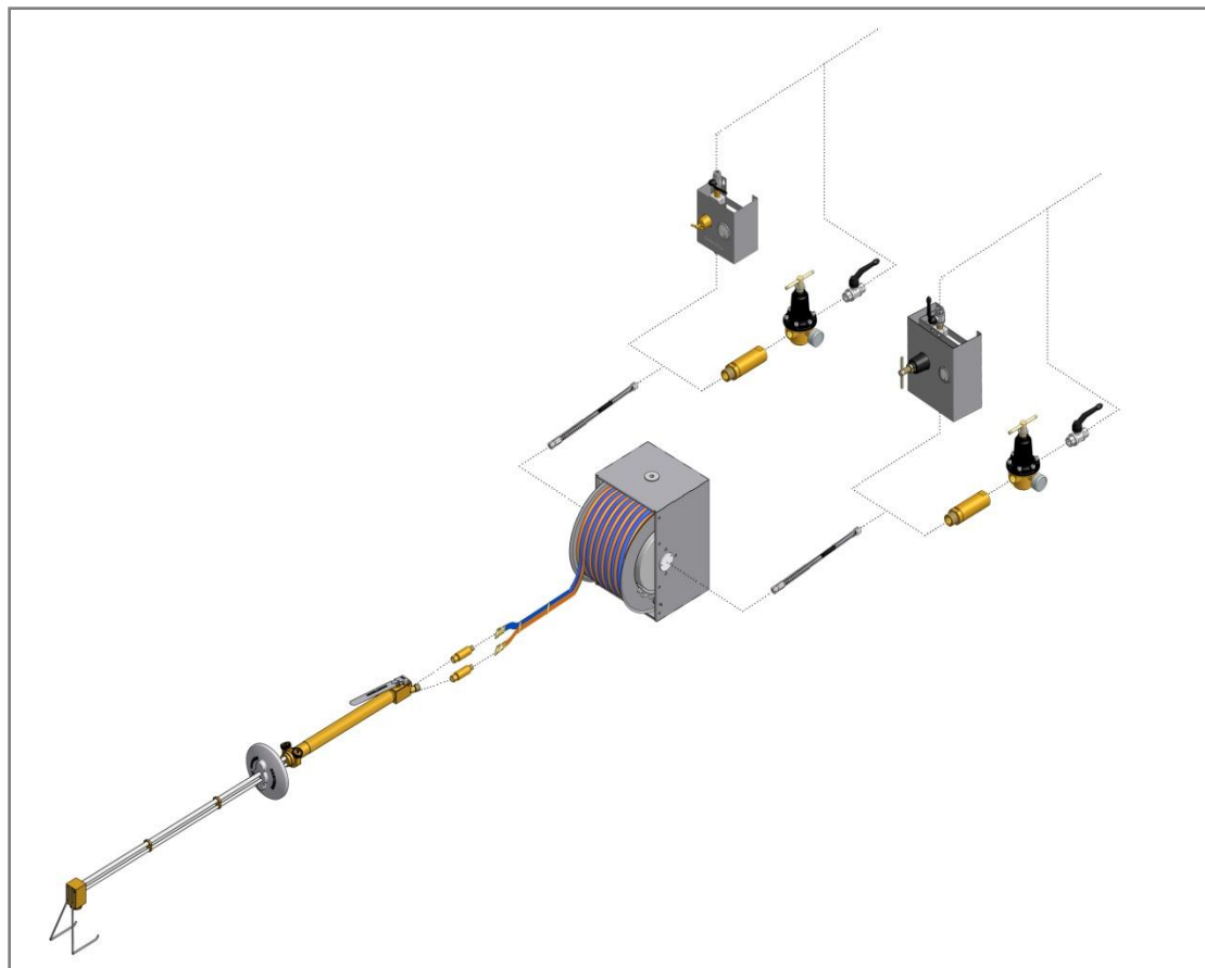
Operating arrangement for quick intervention oxygen-cutting equipment Schema d'impiego per l'attrezzatura ossitaglio pronto intervento
